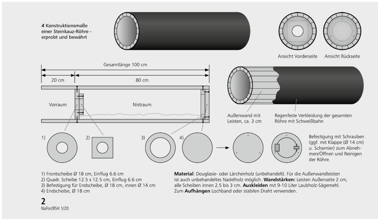
Abbildung 1 Konstruktionsmaße einer Steinkauz-Röhre - erprobt und bewährt [Quelle BSH-Archiv]
